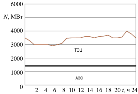
Рис. 4. Суточный график нагрузки ОЭС (зима, ВД, в работе один энергоблок Белорусской АЭС, прогноз)
