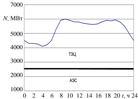
Рис. 3. Суточный график нагрузки ОЭС (зима, РД, в работе один энергоблок Белорусской АЭС, прогноз)
