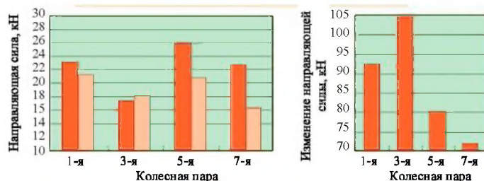
Рис. 2. Направляющая сила и ее изменение при использовании оптимизированной системы: ■ – стандартный профиль; □ – оптимизированный профиль
