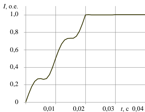
Рис. 4. Переходная характеристика фильтра 1-й гармоники
