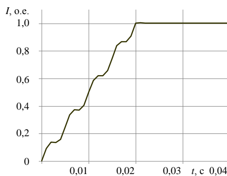
Рис. 5. Переходная характеристика фильтра 2-й гармоники
