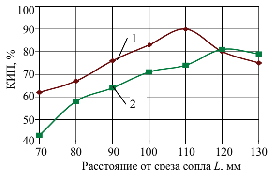
Рис. 2. Зависимость коэффициента использования порошка от дистанции напыления для порошков NiCrAlI с фракцией, мкм: 1 – 40–63; 2 – 63–100 ( I = 550 А, R_{N_2} = 50 л/мин, R_{пор} = 4,5 кг/ч)
