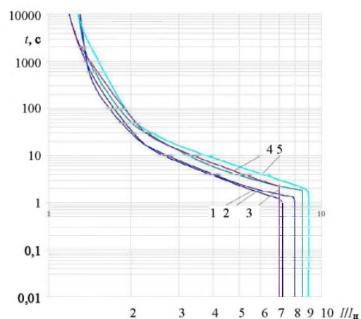
Рис. 7. Экспериментальные ВТХ АВ разных производителей, номинальный ток расцепителей 16 А: 1 – ЭКФ; 2 – ЭТП; 3 – «Полос»; 4 – Moeller; 5 – ИЭК
