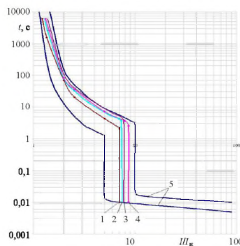
Рис. 3. Экспериментальные ВТХ PL6 производства фирмы Moeller: 1 – I_{н,расц} = 16 А; 2 – 25; 3 – 20; 4 – 32 А; 5 – ВТХ по паспортным данным
