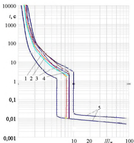
Рис. 5. Экспериментальные ВТХ ВА47-63 производства фирмы «Полос»: 1 – I_{н.расц} = 16 А; 2 – 20; 3 – 32; 4 – 25 А; 5 – ВТХ по паспортным данным
