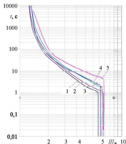
Рис. 8. Экспериментальные ВТХ АВ разных производителей, номинальный ток расцепителей 20 А: 1 – ЭКФ; 2 – ИЭК; 3 – «Полос»; 4 – ЭТП; 5 – Moeller
