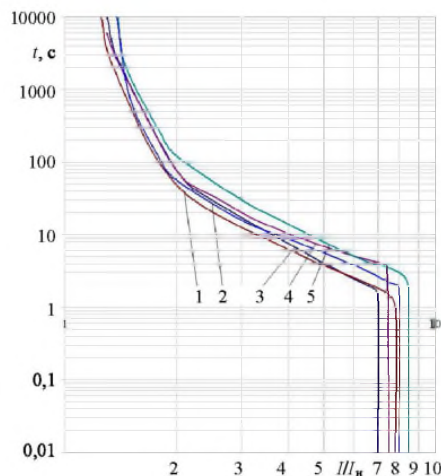
Рис. 9. Экспериментальные ВТХ АВ разных производителей, номинальный ток расцепителей 25 А: 1 – ИЭК; 2 – ЭТП; 3 – ЭКФ; 4 – Moeller, 5 – «Полос»
