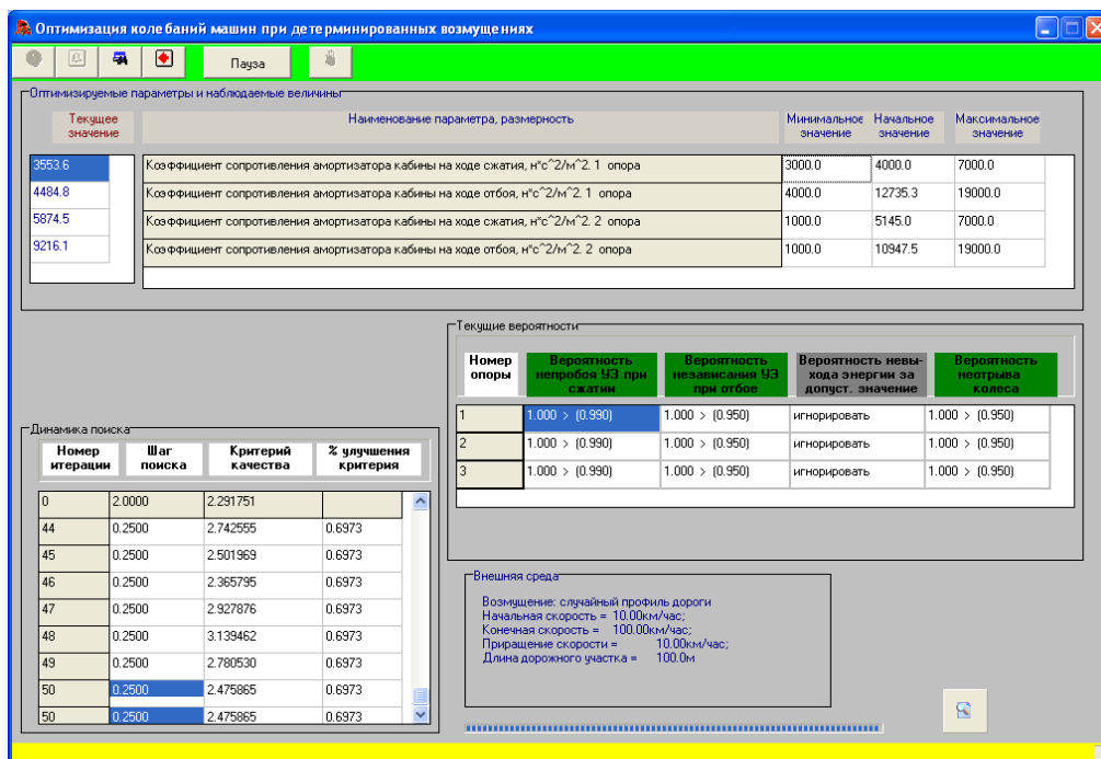
Рис. 8. Окно управления процессом оптимизации
