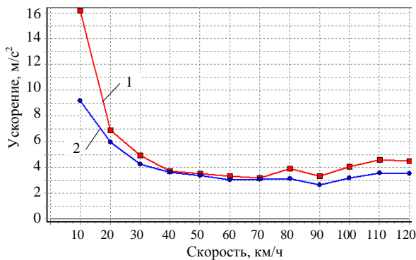
Рис. 9. Зависимость ускорений на полу кабины на месте установки сиденья водителя от скорости при оптимальных параметрах подвески сиденья водителя: 1 – с начальными параметрами; 2 – с оптимальными параметрами
