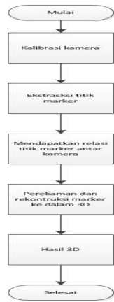
Gambar 8. Flowchart Pengambilan Data pada Motion Capture
