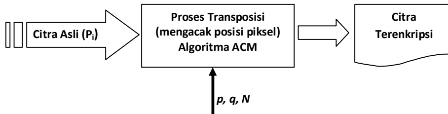
Gambar 1. Bentuk Umum Proses Enkripsi Menggunakan Arnold's Cat Map
