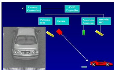
Gambar 4. Ilustrasi kendaraan terdeteksi mendekati sensor pendeteksi RFID sensor pendeteksi kendaraan
