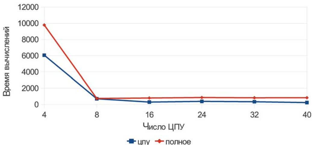
Рис. 8. Зависимость времени расчета энергии ППК (ТАА и 5 ТВБ) от числа ЦПУ
