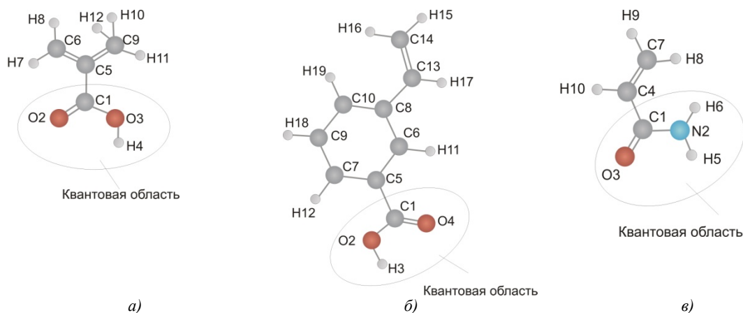
Рис. 3. Функциональные момеры: а) метакриловая кислота; б) мета-винил-бензойная кислота; в) акриламид
