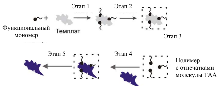
Рис. 1. Этапы процесса получения и применения полимера с отпечатками молекулы ТАА: 1 – получение ППК; 2 – полимеризация; 3 – вымывание темплата из полимера; 4 – селективное извлечение молекул, которые соответствуют сформированным отпечаткам по форме, размеру и наличию функциональных групп, способных взаимодействовать с функциональными группами мономеров; 5 – вымывание выбранных молекул
