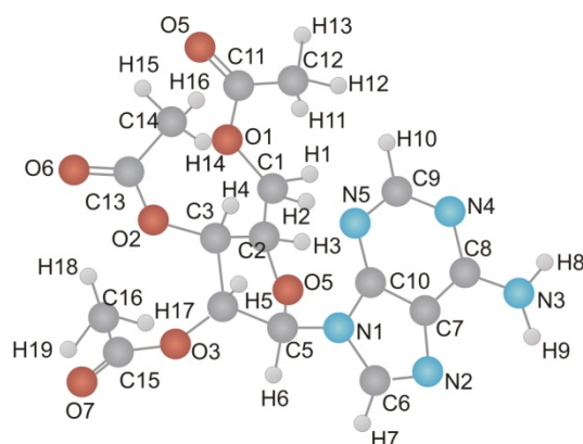
Рис. 2. Молекула ТАА
