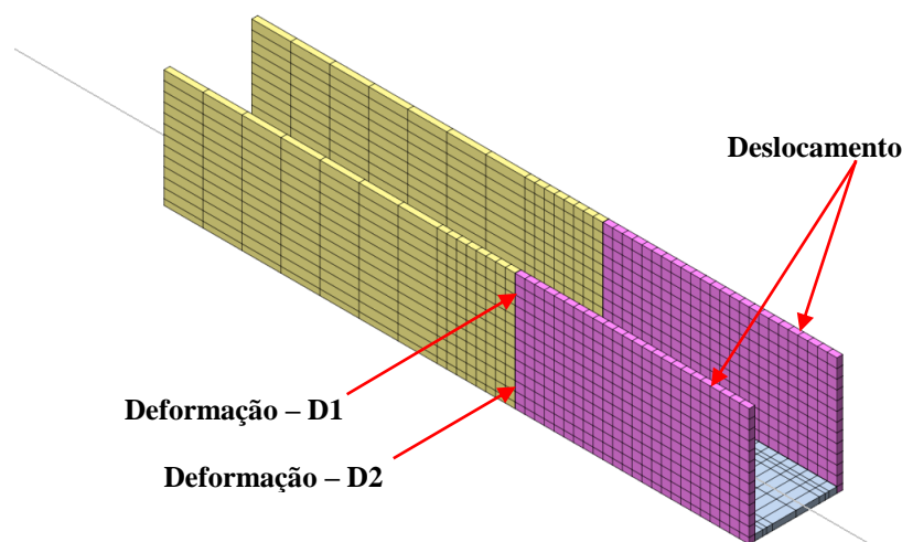
Figura 11. Nós considerados para extrair as deformações e deslocamento nos modelos computacionais.
