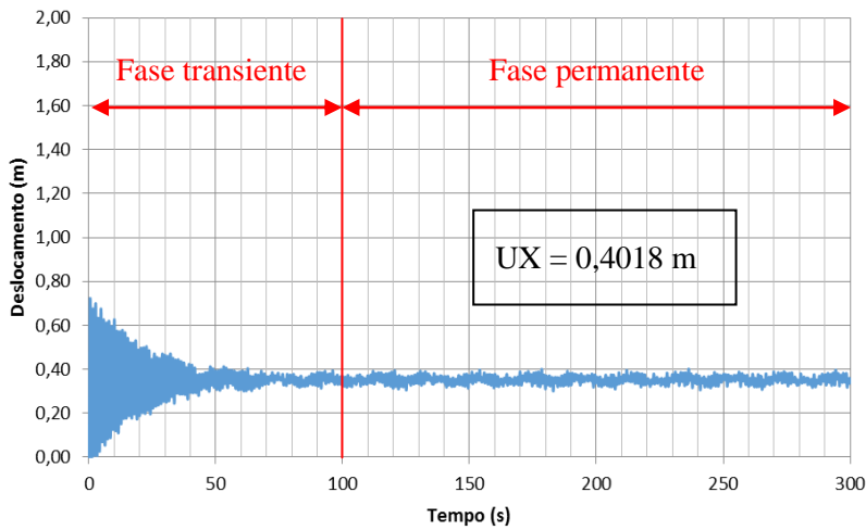
Figura 14. Resposta dinâmica V_0 = 40 m/s; série de carregamento 5
