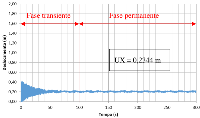
Figura 13. Resposta dinâmica V_0 = 35 m/s; série de carregamento 5
