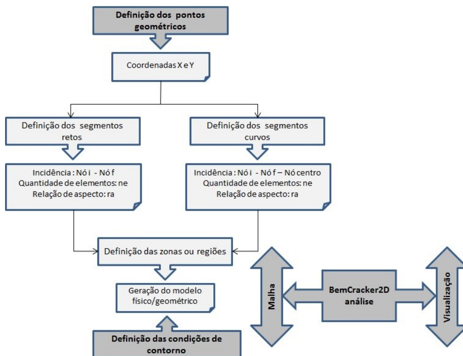
Figura 2 – Hierarquia de funcionalidade da Interface BEMLAB2D.
