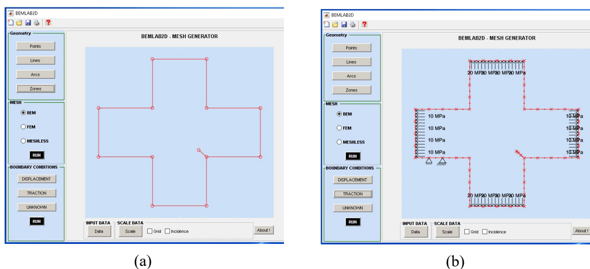
Figura 13. Placa cruciforme trincada: a) Desenho do modelo; b) Malha e condições de contorno.
