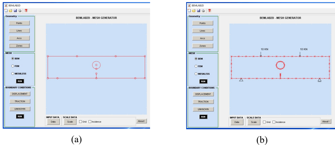
Figura 15. Placa retangular com três furos: a) Modelo problema; b) Modelo gerado pelo BEMLAB2D.
