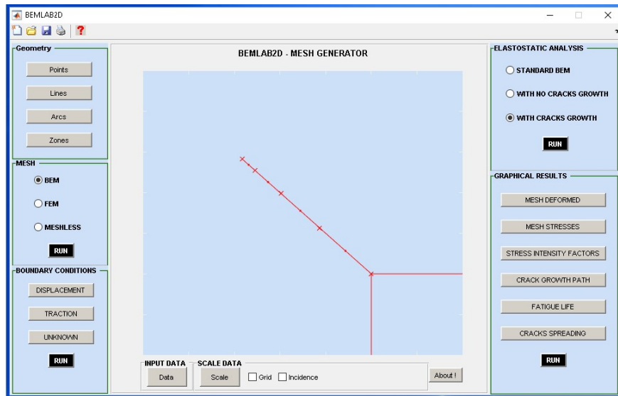
Figura 14. Malha de elementos de contorno gerada pelo BEMLAB2D e detalhe da trinca ampliada.
