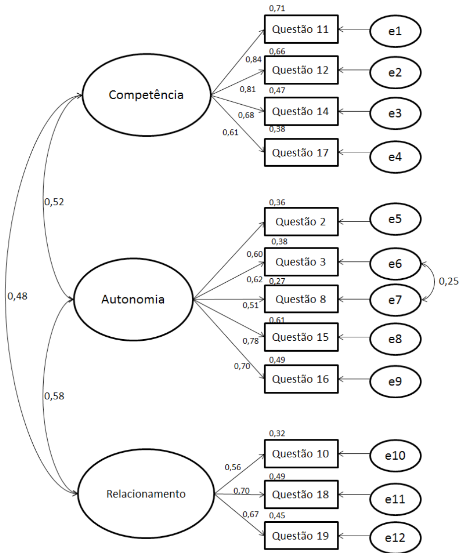
Figura 1. Carga fatorial, intercorrelações entre fatores e erro associado a cada item no modelo de 3 fatores com 12 itens da BNSSS (M4).
