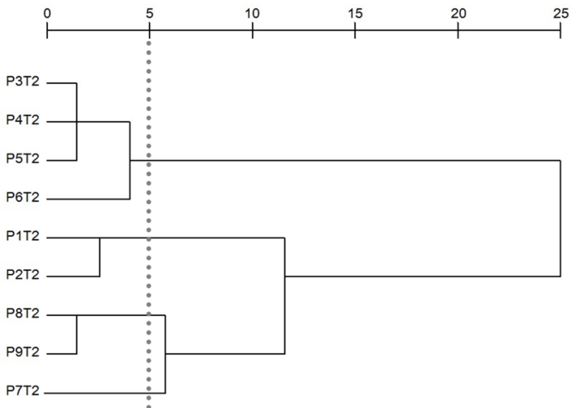
Figura 13– Dendrograma do Transecto 2
