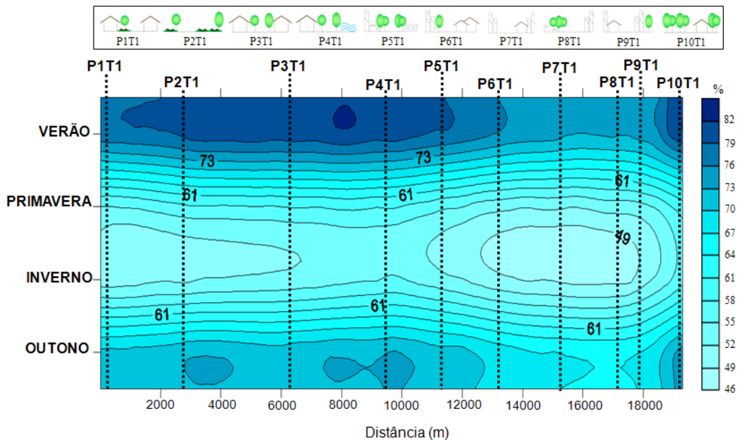
Figura 9– Distribuição da umidade no Transecto 1
