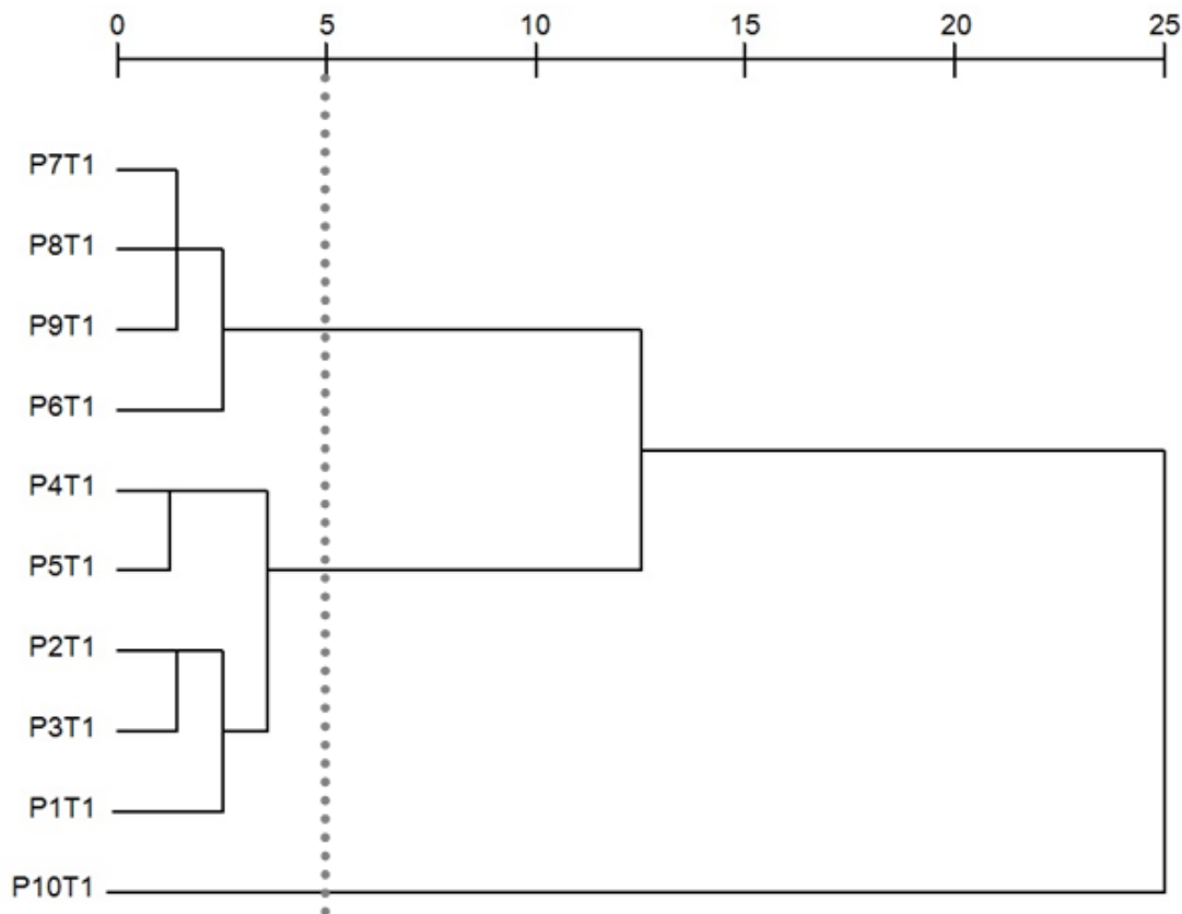
Figura 12– Dendrograma do Transecto 1
