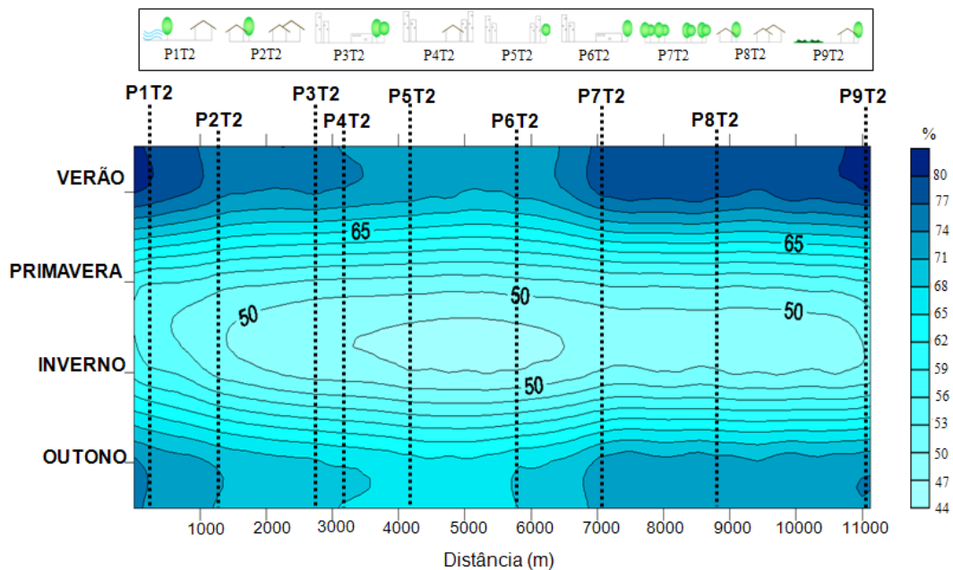
Figura 11– Distribuição da umidade no Transecto 2
