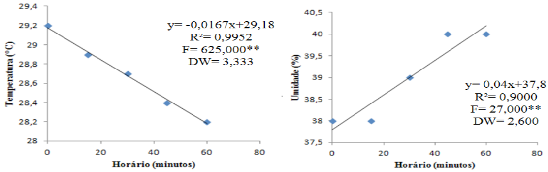
Figura 7–Regressão linear para Transecto 1
