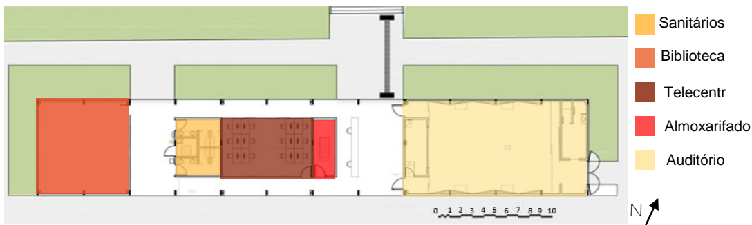
Figura 6. Bloco cultural CEU Professor Samoel Brondi
