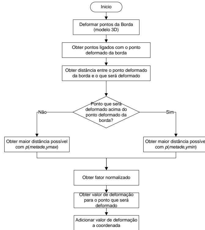
Figura 18. Fluxograma do algoritmo de deformação proposto.
