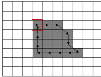
Figura 13. A borda do algoritmo Contour Following após percorrer todo objeto desejado.
