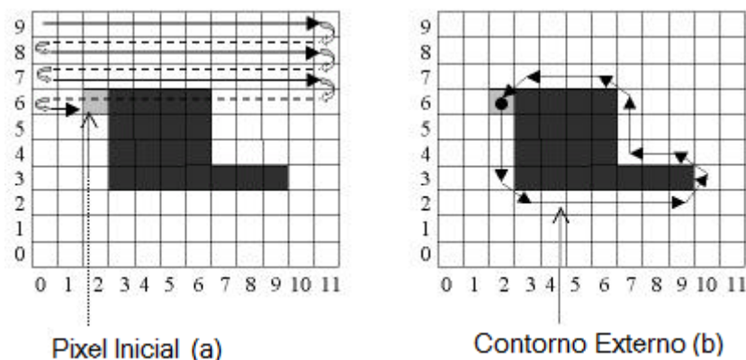
Figura 7. Esquemas ilustrando o algoritmo Contour Following .
