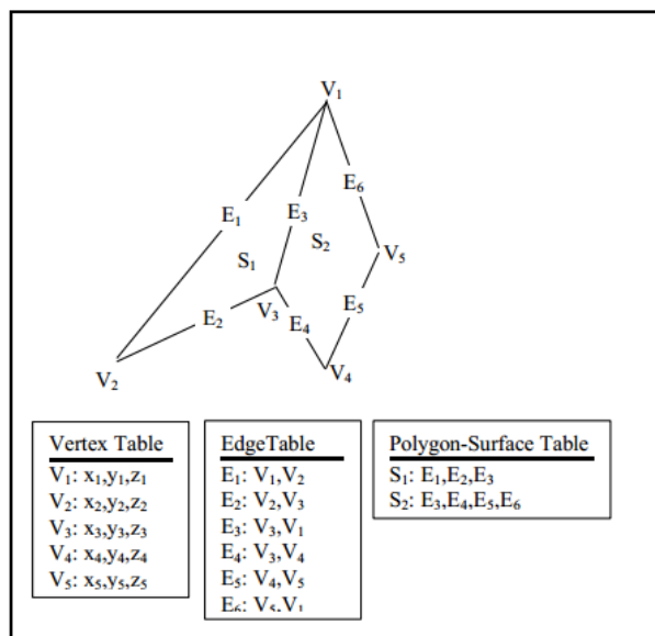
Figura 15. Esquema ilustrando um objeto poligonal.
