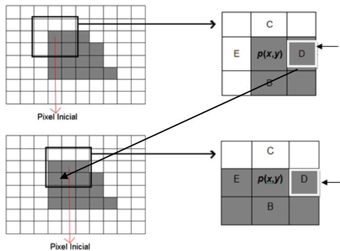
Figura 12. Comportamento do Algoritmo Contour Following .
