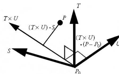
Figura 1. Vetores S, T e U com um ponto registrado no sistema de coordenadas.
