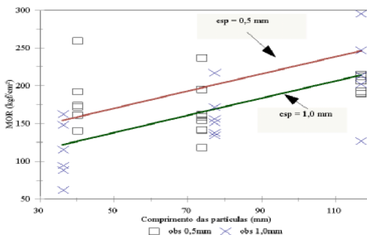
FIGURA 1: MOR observado e estimado em função do comprimento das partículas, para as duas espessuras estudadas.
