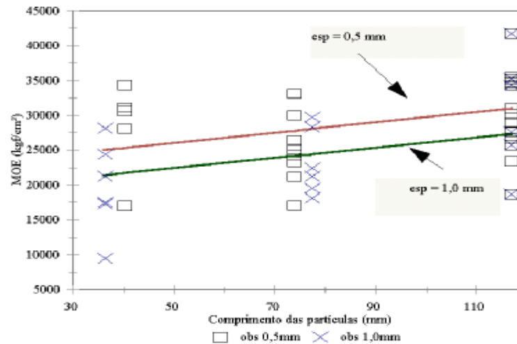
FIGURA 2: MOE observado e estimado em função do comprimento das partículas, para as duas espessuras estudadas.
