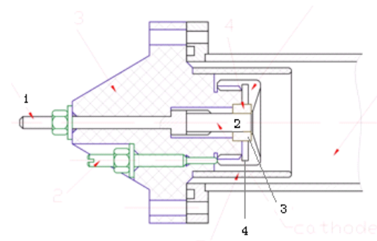
Gambar 2. Susunan sistem elektrode ignitor.
