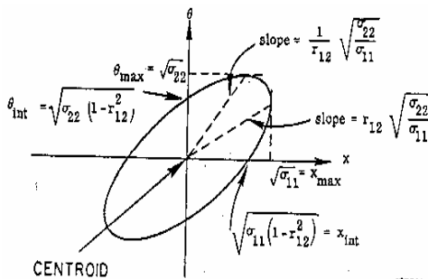
Gambar Elips fase pada bidang (X,X')
