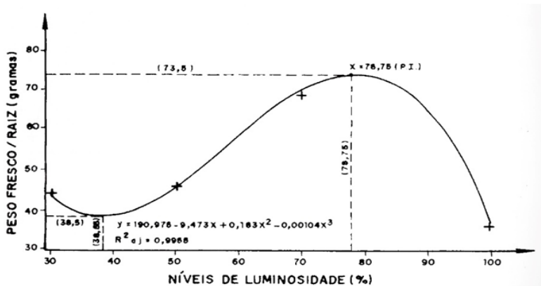
FIGURA 5: Estimativa de massa fresca do sistema radicular em função dos níveis de luminosidade e médias observadas (+).
