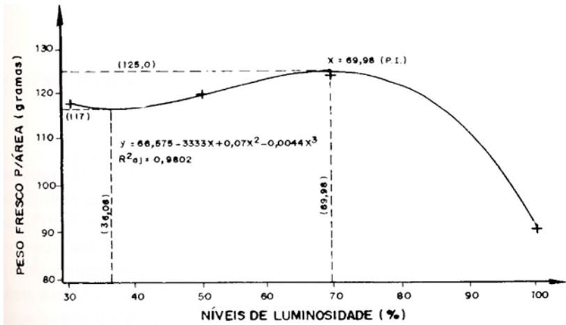
FIGURA 4: Estimativa de massa fresca da parte aérea em função dos níveis de luminosidade e médias observadas (+).
