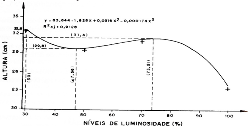
FIGURA 1: Curva ajustada a altura em função da intensidade luminosa e as médias dos níveis de luminosidade (+).
