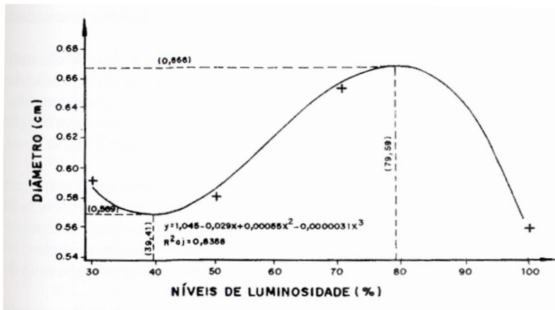
FIGURA 3: Estimativa de massa fresca em função dos níveis de luminosidade, das médias dos níveis e da luminosidade (+).
