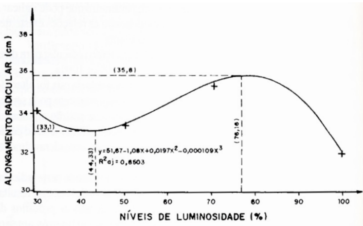
FIGURA 8: Curva ajustada do alongamento radicular em função da intensidade luminosa e as médias observadas (+).
