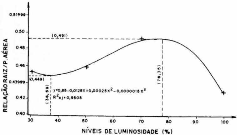
FIGURA 7: Curva ajustada da relação raiz/parte aérea em função da intensidade luminosa e as médias dos níveis de luminosidade (+).
