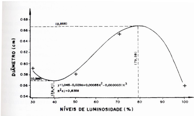
FIGURA 2: Curva ajustada do diâmetro do colo em função da intensidade luminosa e as médias dos diferentes níveis de luminosidade (+). FIGURE 2: Adjusted curve of the diameter of the neck as a function of the luminous intensity and the means of the different levels of luminosity (+).
