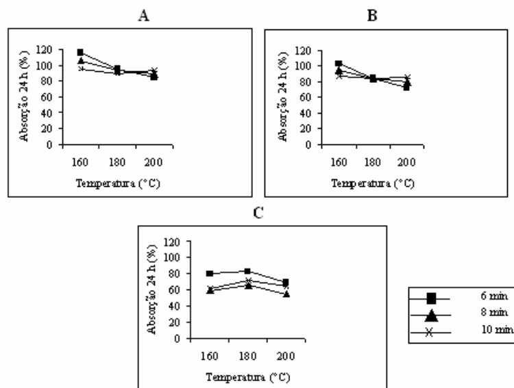
FIGURA 4: Cortes nas superfícies de resposta ajustada para a variável dependente absorção de água 24 h para os teores de resina 3% (A), 4,5% (B) e 6% (C).
