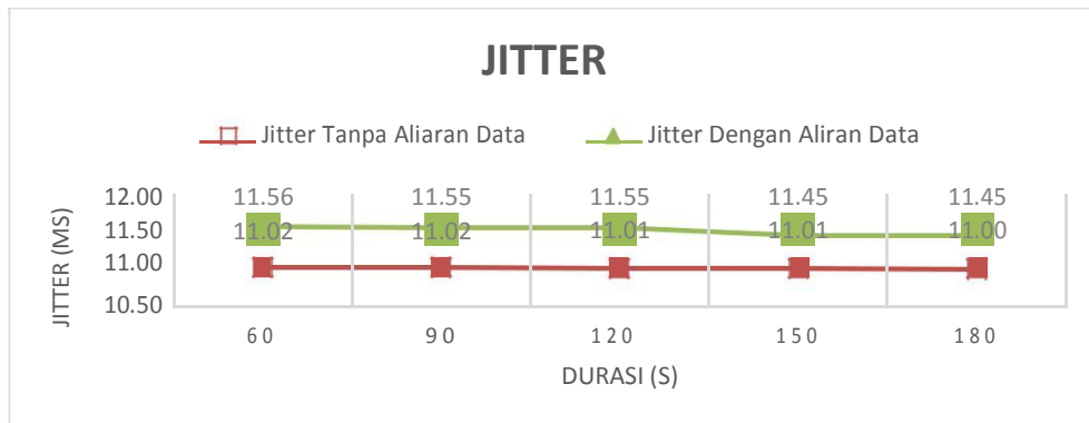
Gambar 3. Grafik Jitter Layanan VoIP
