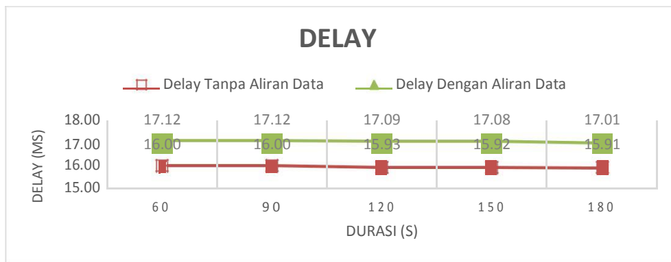
Gambar 2. Grafik Delay Layanan VoIP
