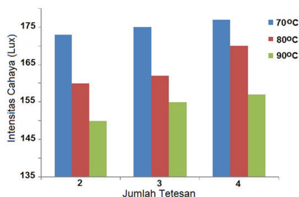
Gambar 1. Grafik hasil pengukuran intensitas cahaya
