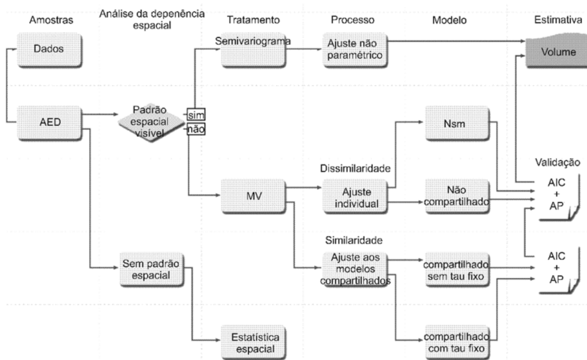
FIGURA 2: Fluxograma da metodologia de análise dos dados, ajuste e seleção dos modelos.
