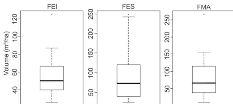
FIGURA 3: Gráfico Box-plot da dispersão do volume (m 3 ha -1 ) nas áreas de FEI = floresta em estágio inicial; FES = floresta em estágio secundário; FMA = floresta madura.
