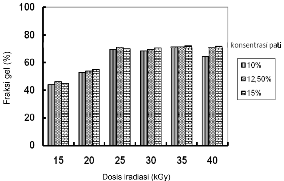
Gambar 1. Fraksi gel hidrogel PVP-pati pada berbagai tingkat dosis iradiasi
