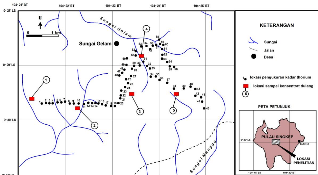
Gambar 2. Peta lintasan pengukuran kadar torium dan lokasi sampel konsentrat dulang di kawasan laterit bauksit.
