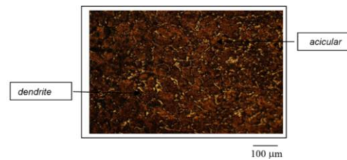
Gambar 1. Mikrograf ingot paduan Zr- 0,3%Nb-0,5%Fe-0,5%Cr
