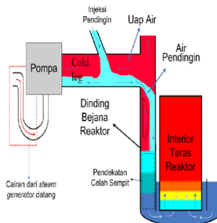
Gambar 1. Skema pendekatan kanal sempit pada saat injeksi temperatur dan tekanan rendah
