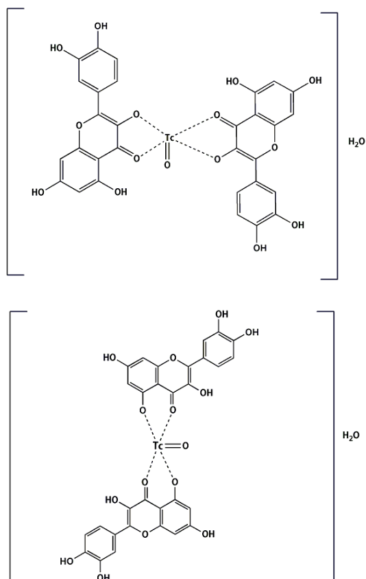
Gambar 2. Prediksi struktur kompleks ^{99m}\text{Tc} -kuersetin (24)
