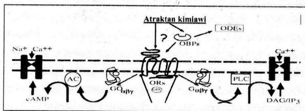
Gambar 3. Mekanisme penghidu pada nyamuk, gambar skematik komponen intraseluler jalur transduksi sinyal olfaktorius. Protein reseptor bau penghidu (OR) ada didalam dendrite ORN yang berinteraksi langsung dengan bau atau alternatifnya membentuk kompleks senyawa protein pengikat bau (atraktan). 20
