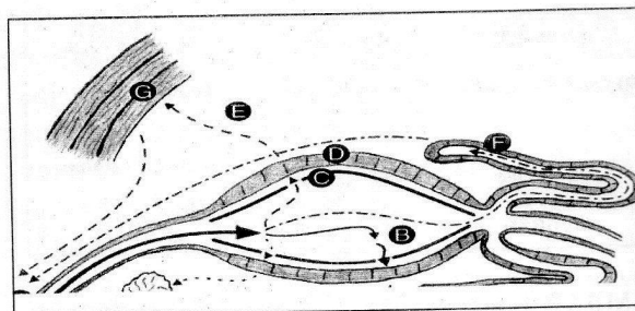
Gambar 2. Rute migrasi dan tempat-tempat perkembangan virus, parasit malaria dan cacic filarial dalam tubuh nyamuk. Tempat perkembangan ditandai dengan huruf A sampai H, rute migrasi diwakili garis. Setelah nyamuk mengisap darah (A), seluruh ben pathogen masuk ke usus tengah/midgut (B). Viru diwakili tanda garis tidak terputus) masuk samp kedalam sel epitel usus tengah/midgut (D), selanjutn berturut-turut mengalami replikasi, keluar dari sel d melintasi hemolymph terisi hemocoel (E) sampai kelenjar liur nyamuk (H) untuk kembali mengalar replikasi dan menetap disana siap untuk 'diinjeksika pada inang vertebrata. Parsit malaria (ditandai deng garis terputus) tetap berada dalam usus tengah/midg selama beberapa jam sambil mengalami syngami d membentuk ookinet sebelum bermigrasi melintasi matri peritropik (C). Selanjutnya setelah melintasi epitel us tengah/midgut, parasit malaria berada diantara lapis epitel dan membrane basal usus tengah/midgut .ooki menjalani sporogoni untuk menghasilkan sporozoit. Sa matang, sporozoit merusak ookista, melintasi hemoco dan berpenetrasi ke kelenjar liur, siap menung diinjeksikan ke inang. Sedangkan pada cacic filari yang menyebabkan penyakit pada manusia (ditand dengan garis terputus) dan pada jantung anjing (ga terputus dengan titik diantaranya) terisap nyamuk, caci
