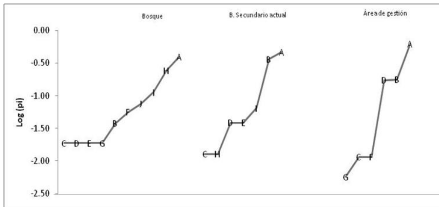
FIGURA 2 Curvas de rango-abundancias de la comunidad de Anolis en tres coberturas vegetales en la selva pluvial tropical en la zona centro del Chocó
