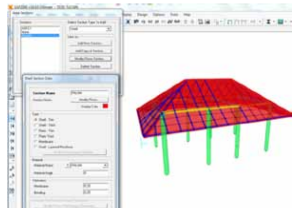
Figura 18. Propiedades geométricas de la cubierta. Fuente: Sap2000
