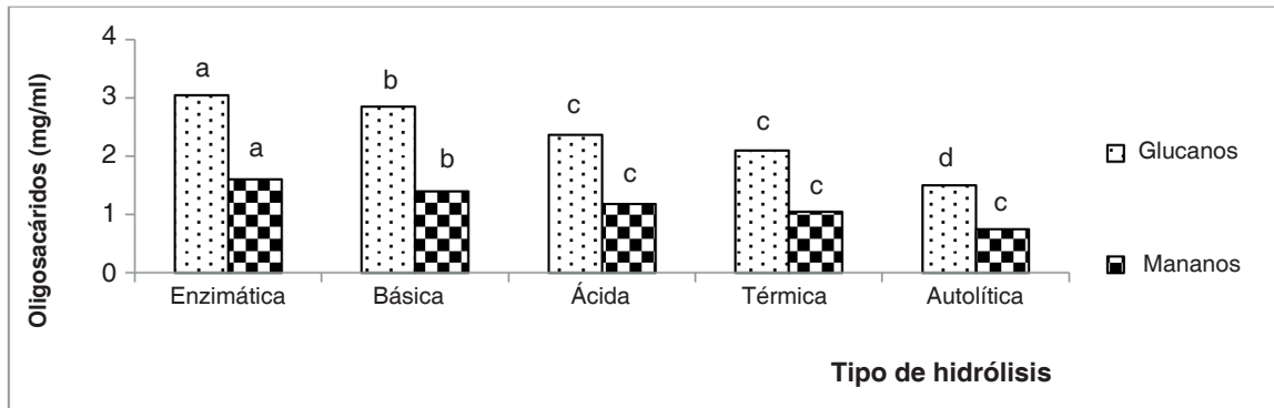
Figura 2. Contenidos de glucanos y mananos según la hidrólisis utilizada. a,b,c,d Letras diferentes entre tipos de hidrólisis difieren para P < 0.01 (Duncan, 1955)
