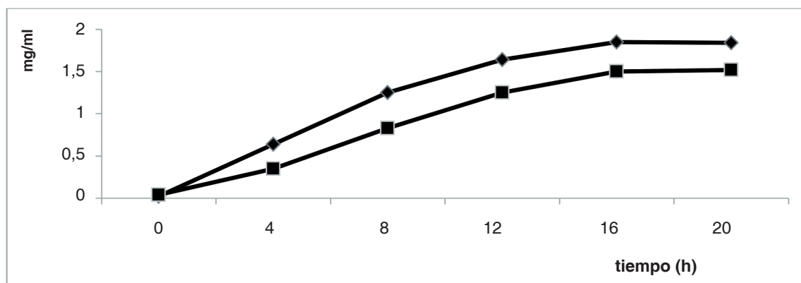
Figura 5. Comportamiento en el tiempo de los contenidos de oligosacáridos de glucanos y de mananos de hidrólisis enzimática de pared de S. cerevisiae .
