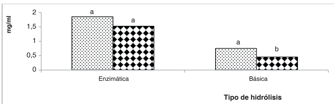
Figura 4. Contenidos oligosacáridos de glucanos y mananos de la hidrólisis enzimática y básica de paredes celulares aisladas de Saccharomyces cerevisiae . a,b Letras diferentes entre tipos de hidrólisis difieren para P < 0.001 (Duncan, 1955).
