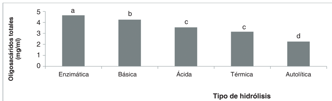
Figura 1. Valores promedios de oligosacáridos totales obtenidos de diferentes tipos de hidrólisis. a,b,c,d Letras diferentes entre tipos de hidrólisis difieren para P<0.05 (Duncan, 1955) P<0.01
