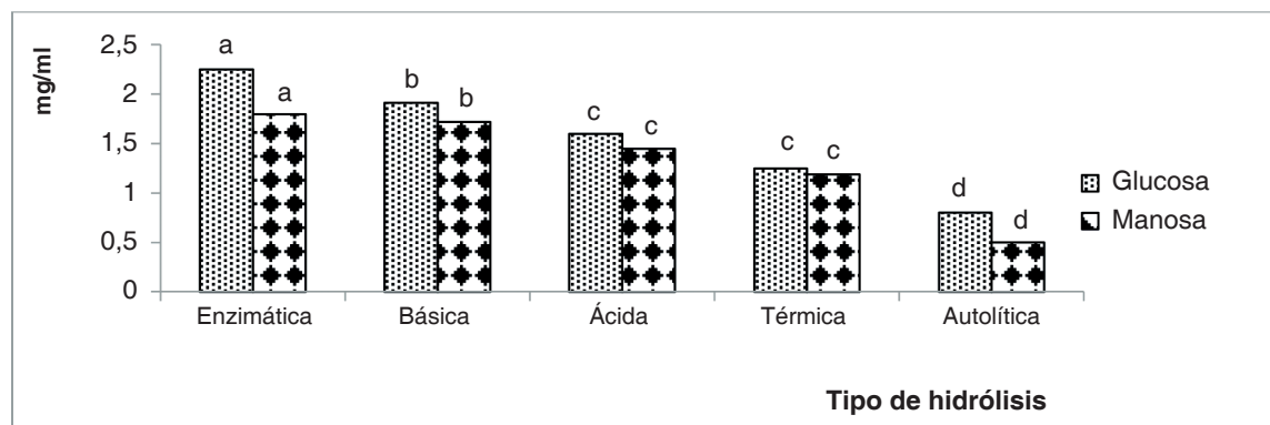
Figura 3. Contenidos de glucosa y manosa en mg/ml según tipos de hidrólisis. a,b,c,d Letras diferentes entre tipos de hidrólisis difieren para P < 0.01 (Duncan, 1955).
