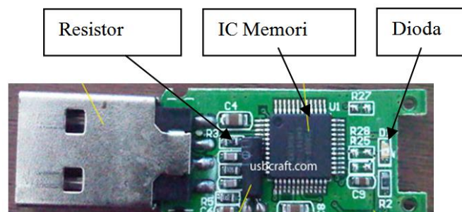
Gambar 1. Bagian-bagian flashdisk
