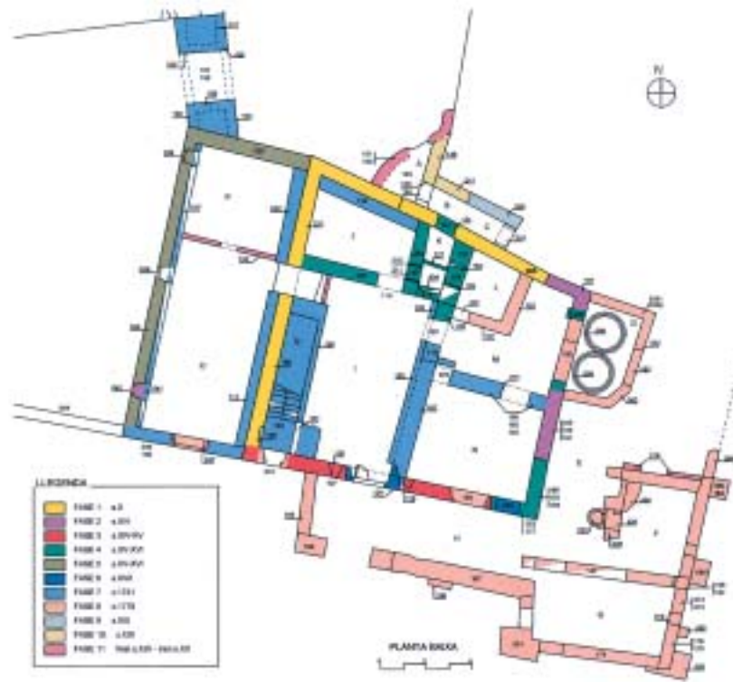
Fig.14. Planta de la casa parroquial de Castellnou de Bages con indicación de la cronología de las diferentes estructuras, 1998
