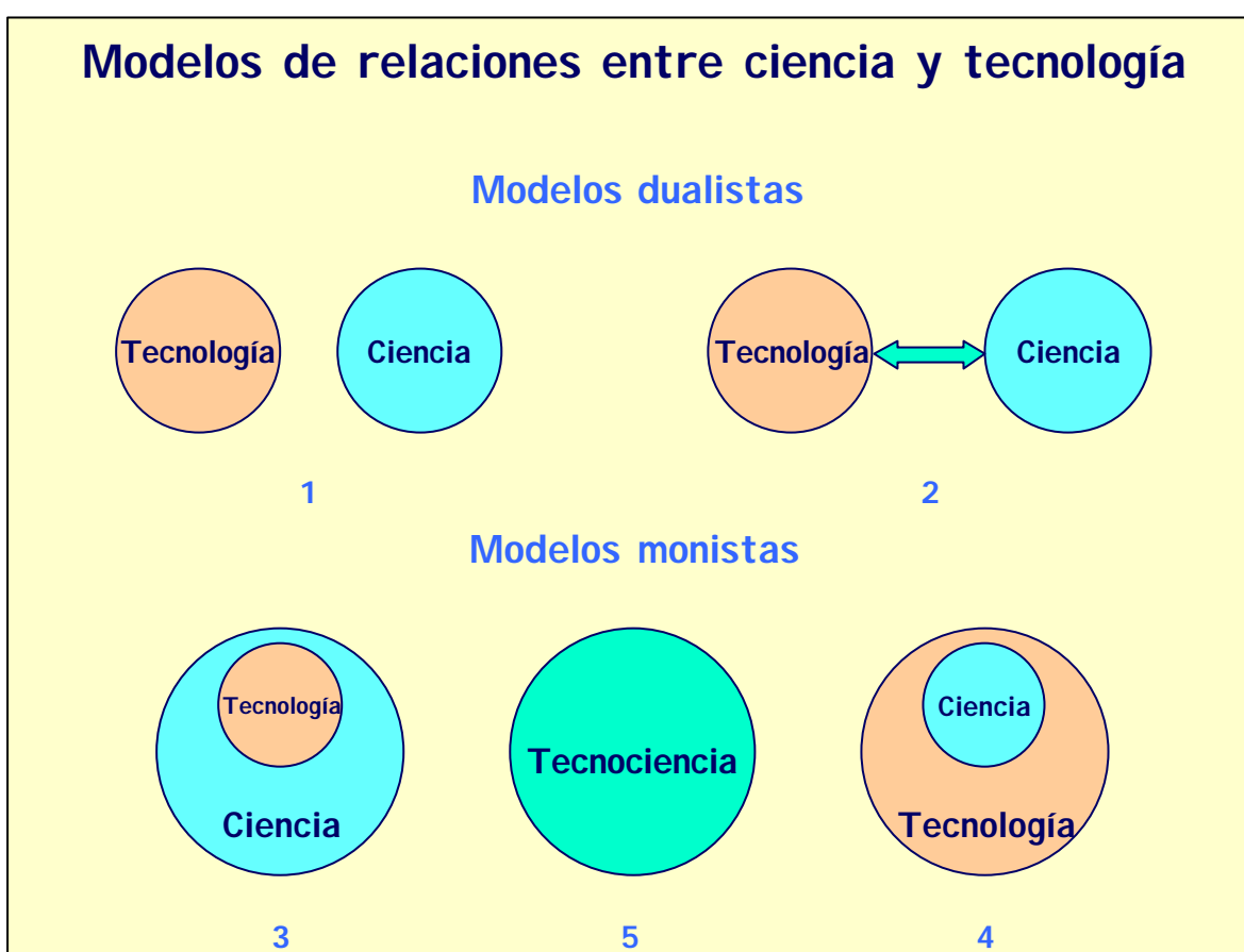
Figura 3.- Esquemas de cinco modelos de relaciones entre ciencia y tecnología.
