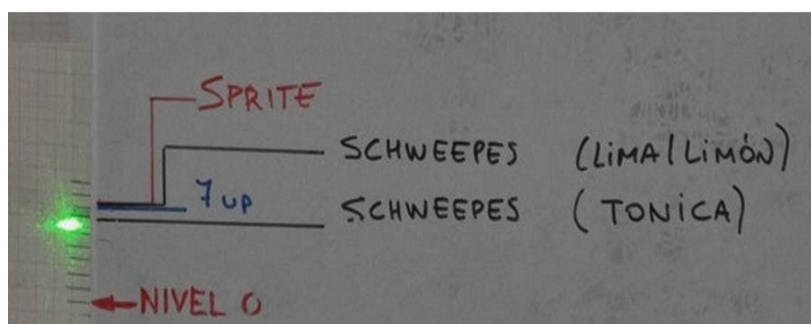
Figura 8. Desviaciones sufridas por el haz para las distintas gaseosas.
