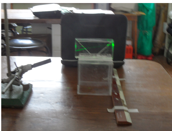
Figura 5. Fotografía del refractómetro, en ella se observan las desviaciones que experimenta el haz de luz al atravesar diferentes medios.
