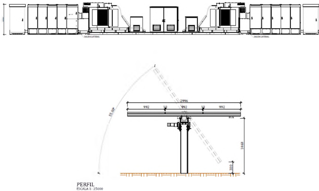
Gráfico Nº2 Centro de Inversores y estructura de seguidores solares.
