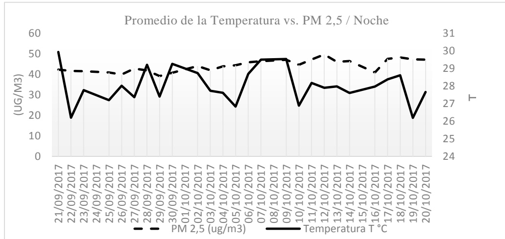
Figura 4. Medida promedio de la Temperatura y la concentración de PM2,5 para las franjas: Día, tarde y noche
