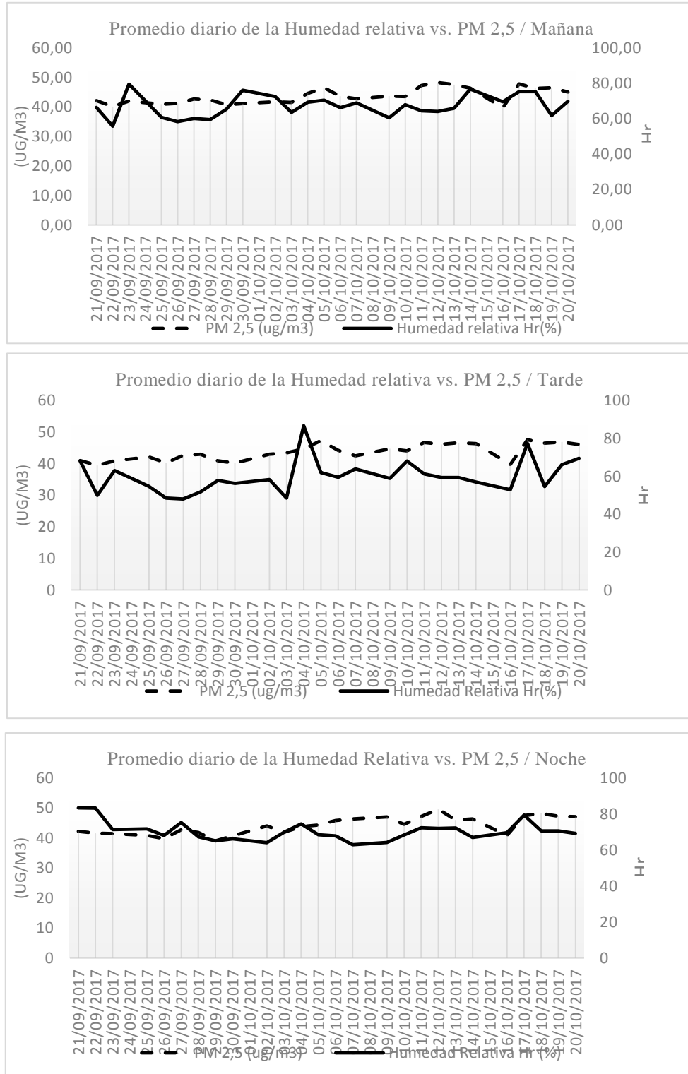
Figura 2. Medida de PM2.5 y COV para las franjas: Día, tarde y noche
