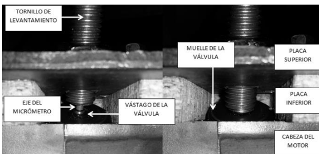
Figura. 5. Acoplamiento de válvula y sistema de levantamiento y medición
