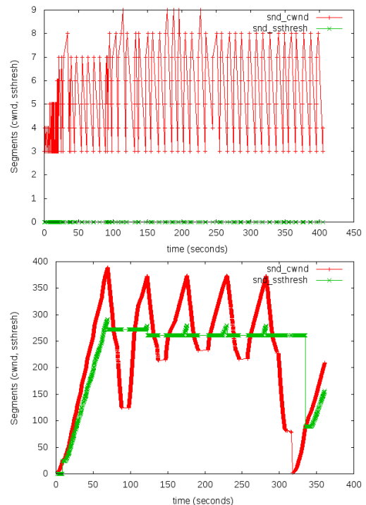
Fig. 8. Ventana de congestión del servidor en transferencia de un archivo de 10 MB desde la VSAT con el acelerador TCP activado (arriba) y desactivado (abajo).
