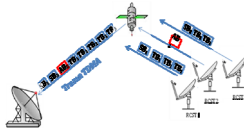
Fig. 2. Esquema de acceso al medio para redes VSAT. Dirección RCST – Central.
