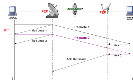
Fig. 3. Topología para el Acelerador TCP
