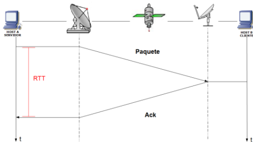
Fig. 1. Impacto del enlace satelital sobre el Tiempo de Ida y Vuelta (TIV)
