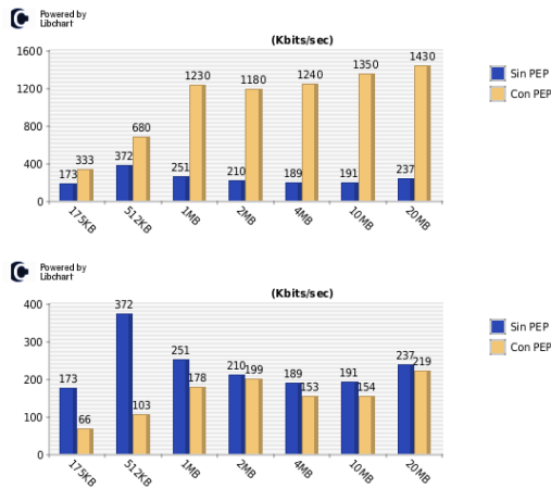
Fig. 6. Resultados prueba de rendimiento (R) para el periodo de tráfico moderado, arriba cuando los datos se transmiten desde un Servidor en la Internet, abajo cuando los datos se transmiten desde una Terminal.
