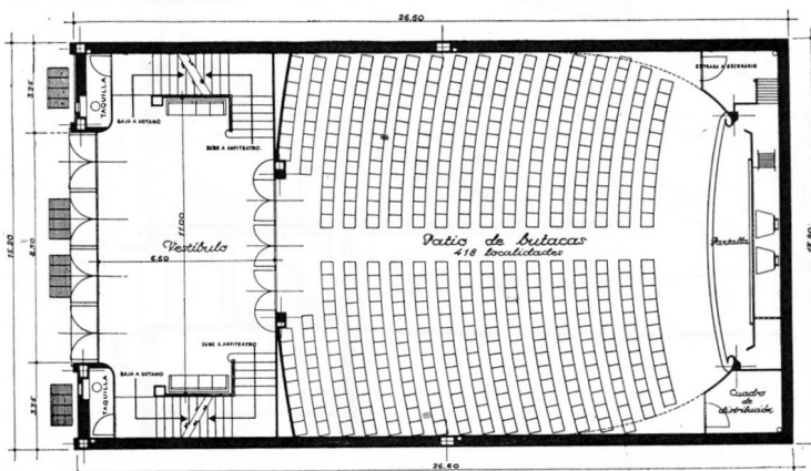
Planta del patio de butacas
