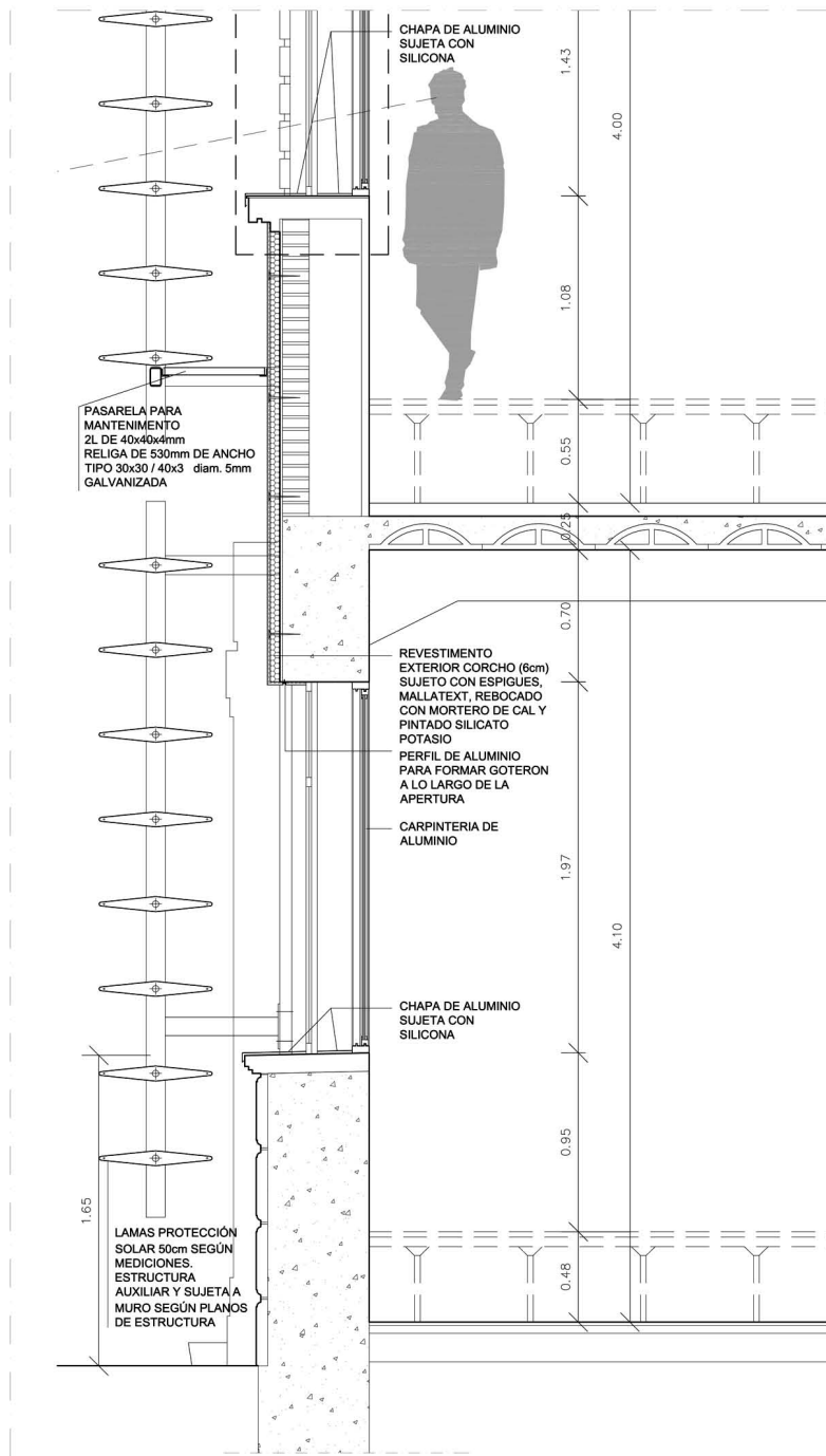
SECCIÓN FACHADA EXTERIOR
