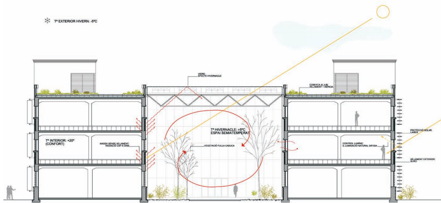
ESQUEMA BIOCLIMÁTIC COMPORTAMENT TÈRMIC HIPÒTESI D'INVERN e. 1/150
