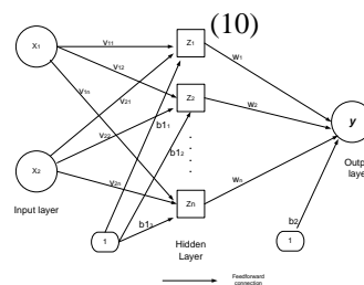
Gambar 7. Arsitektur jaringan propagasi balik.
