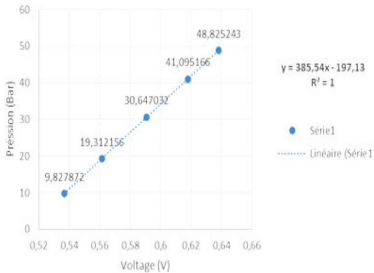
Figure 4: Kit de mesure de pénétromètre vertical muni de capteur électronique de mesure de pression et de système d'acquisition (gauche) et courbe de calibration de force de pénétration Bar = f(V) (droite)
