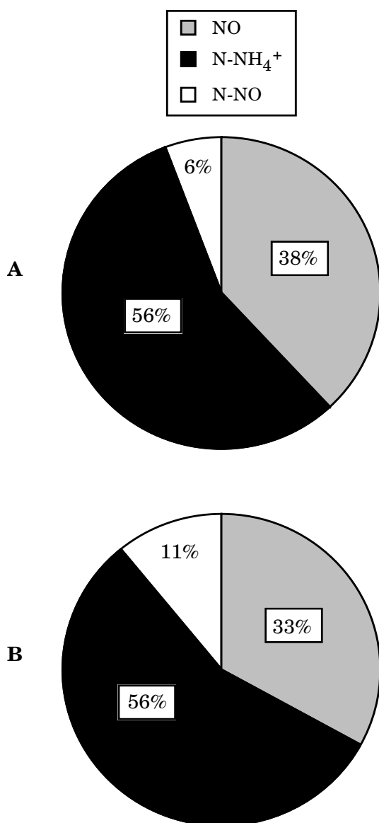
Figure 2. Pourcentage des différentes fractions d'azote au niveau de l'influent (A) et de l'effluent (B) du bassin d'élevage du poisson (NO = N organique, N-NO = forme oxydée de N)
