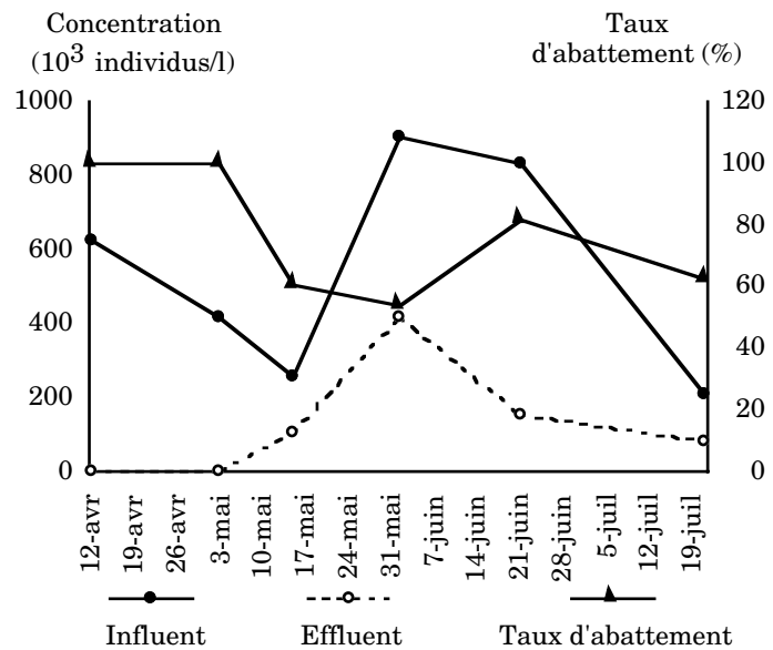
Figure 5. Taux d'abattement et concentration en zooplancton au niveau de l'influent et de l'effluent du bassin d'élevage
