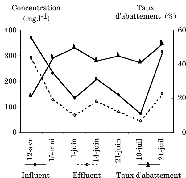
Figure 3. Taux d'abattement et concentration en matières en suspension au niveau de l'influent et de l'effluent du bassin d'élevage
