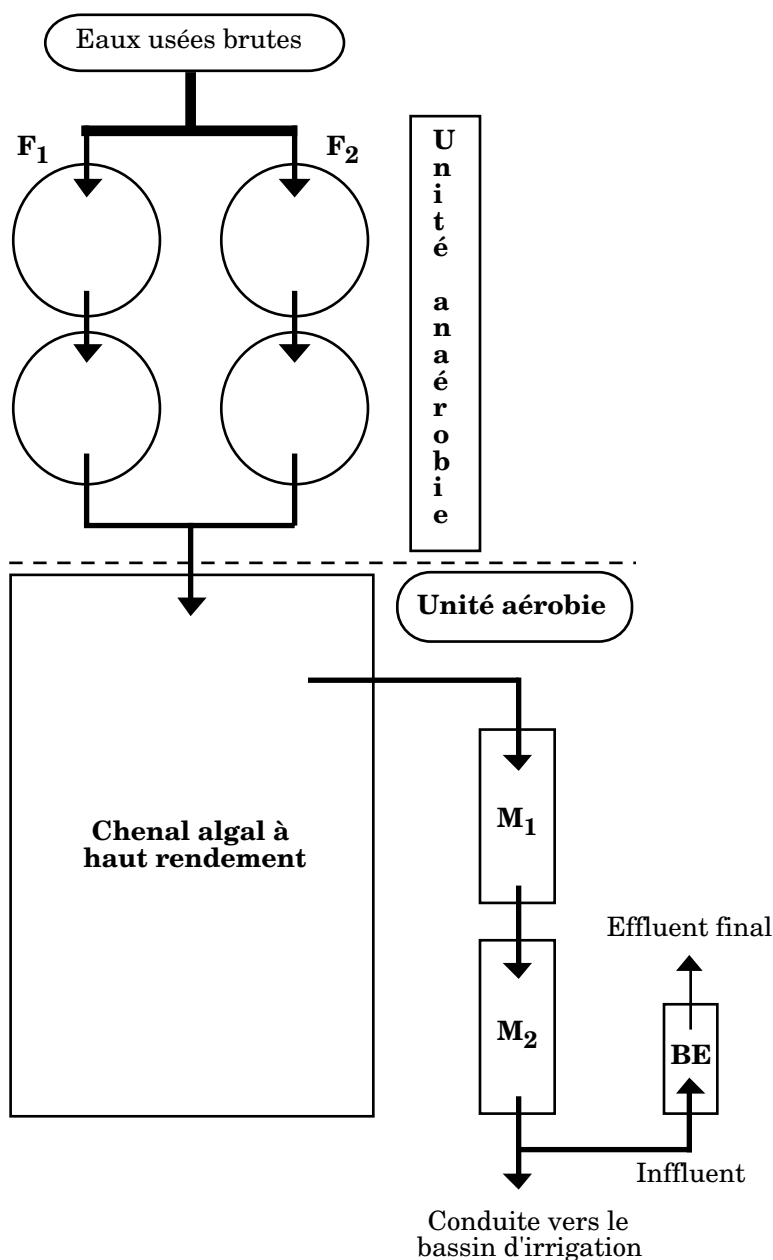
Figure 1. Schéma de l'unité de traitement des eaux usées et du bassin d'élevage de carpes à la station d'épuration de l'IAV Hassan II (Rabat) F 1 & F 2 : Filières anaérobies; M 1 & M 2 : Bassins de maturation; BE: bassin d'élevage de carpes
