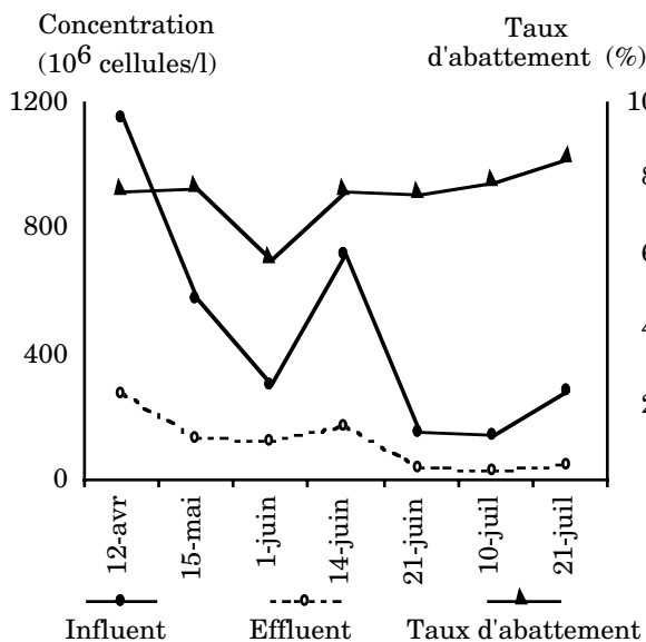
Figure 4. Taux d'abattement et concentration en phytoplancton au niveau de l'influent et de l'effluent du bassin d'élevage
