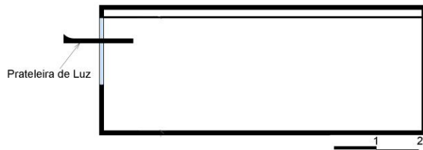
Figura 1: Corte transversal da sala com prateleiras de luz interna e externa. Fonte: Elaboração própria.
