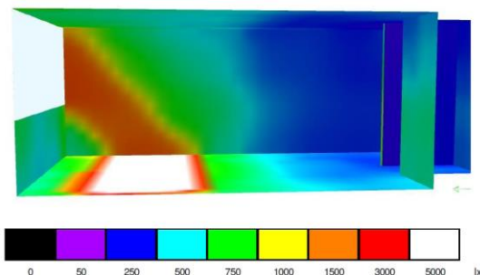
Figura 4: Simulao em cores falsas da sala Norte, sem prateleiras de luz, no solsticio de inverno s 12h. Fonte: Elaborao propria.
