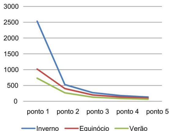
Figura 6: Grafico de distribuio das iluminncias medias da sala Norte sem prateleiras de luz. Fonte: Elaborao propria.
