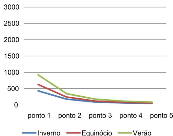
Figura 7: Grafico de distribuio das iluminncias medias da sala Sul sem prateleiras de luz. Fonte: Elaborao propria.
