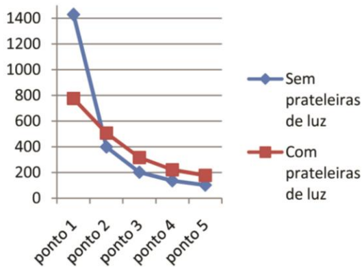
Figura 14: Média das iluminâncias da sala Norte. Fonte: Elaboração própria.
