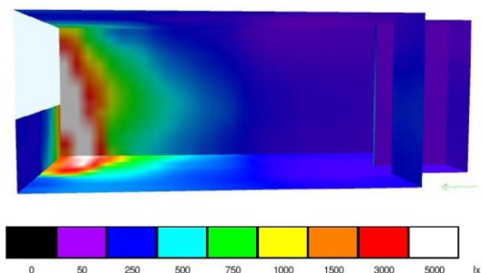
Figura 5: Simulao em cores falsas da sala Sul, sem prateleiras de luz, no solsticio de vero s 8h. Fonte: Elaborao propria.
