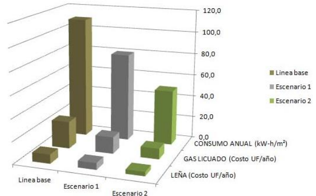
Figura 8: Consumos energéticos por calefacción. Fuente: Elaboración Propia Figure 8: Heating energy consumption. Source: Own Elaboration.
