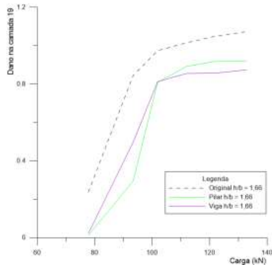
Figura 20 - Avaliação da evolução do dano quando a relação h/b = 1,66 . Fonte: Elaborado pelos autores
